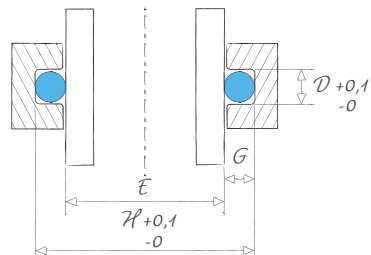
Alésage
