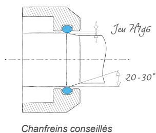
Montage alésage
