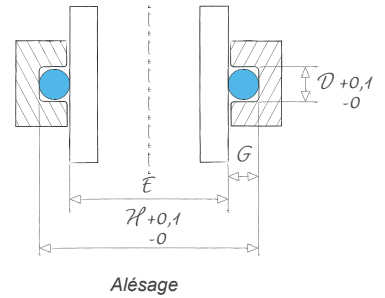
Piston
